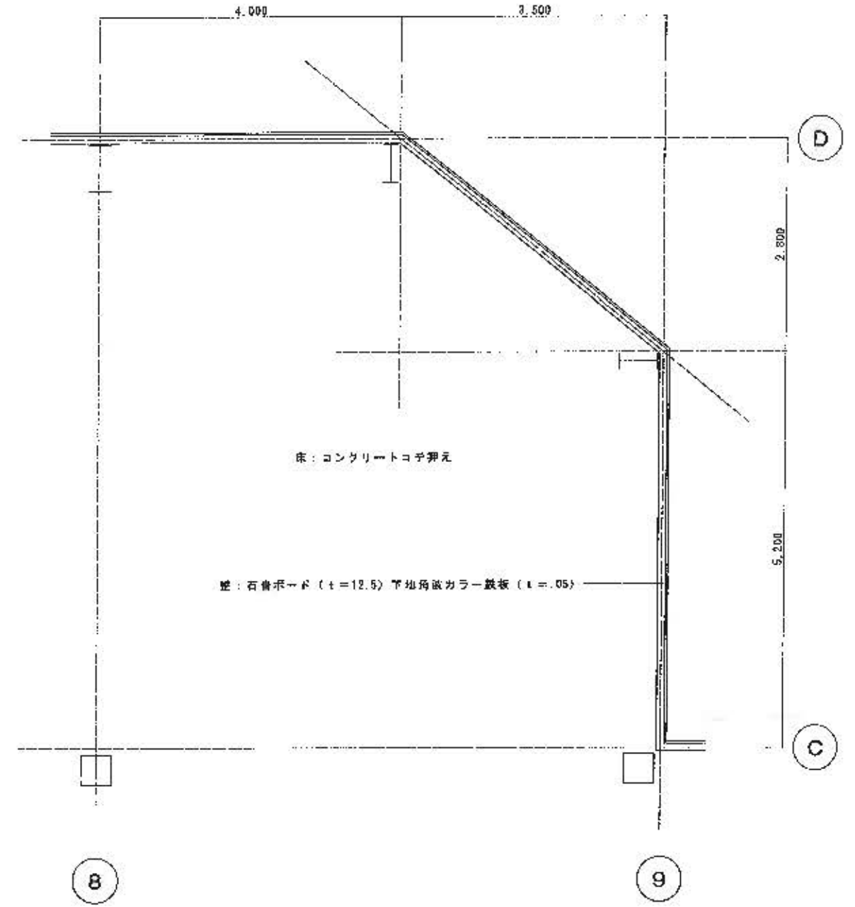
1・2階改造後平面詳細図 S=1:50
