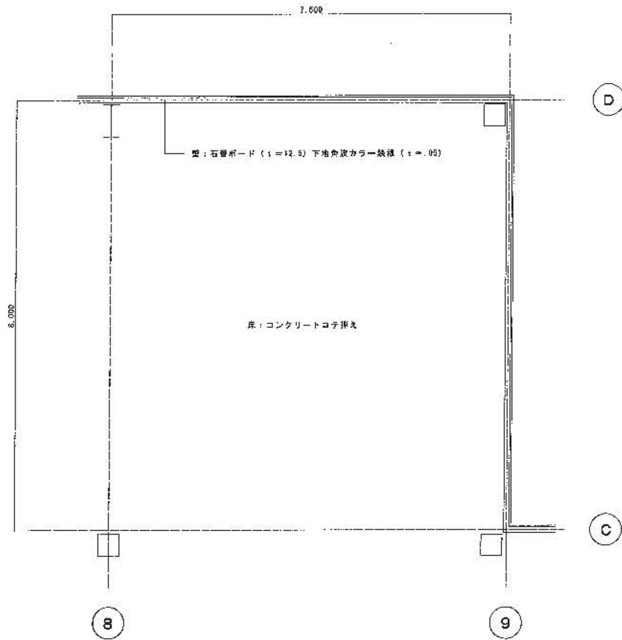
1・2階改造前平面詳細図 S=1:50
