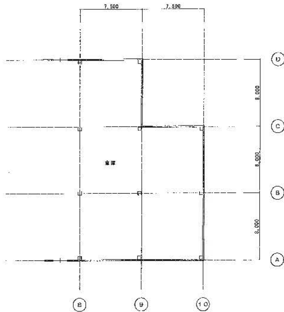
改造前 1, 2 階平面図 S = 1/200
