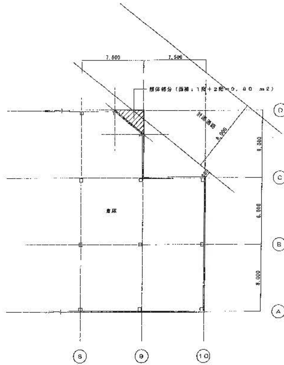
改造後 1, 2 階平面図 S = 1/200
