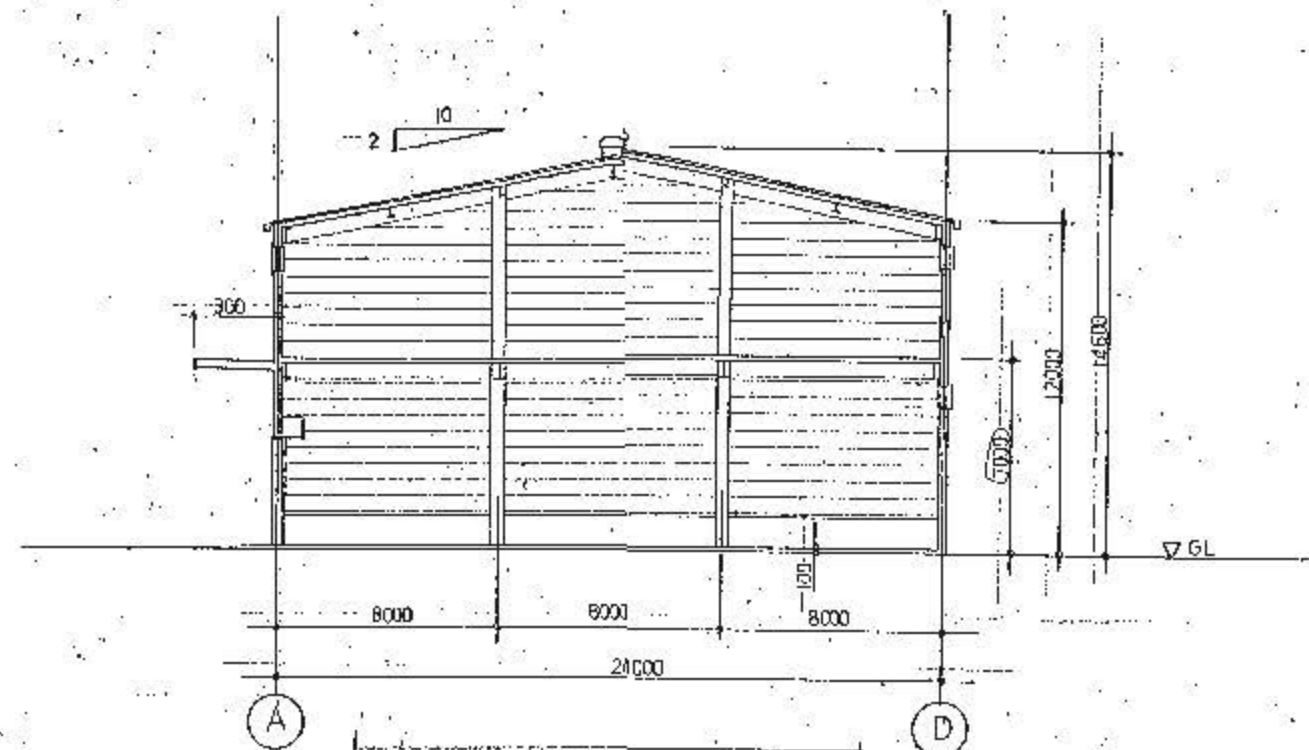
断面図 S=1:200
